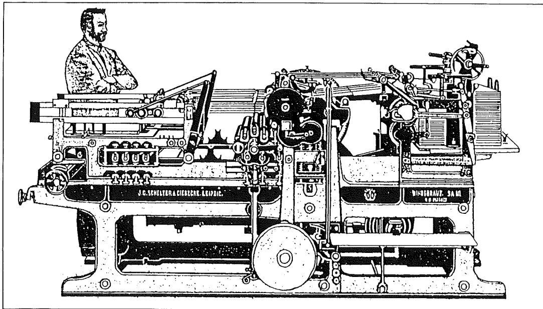
□ Fig. 4. Tussjtegning av den «Windsbraut-toturs-hurtigpresse» som boktrykker Chr. H. Knudsen anskaffet i 1918 til bruk for trykning av frimerker og portomerker m.m.
