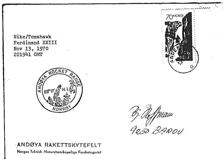
□ Fig. C: Typisk astro-brev som beskriver oppskyting av en rakett fra Andøya Rakettskytefelt. Brevet er korrekt stemplet på samme dag som oppskytingen, og bærer alle nødvendige data om sted, tid, klokkeslett og type rakett. Det offisielle si-destempelet er et pluss for brevet.
