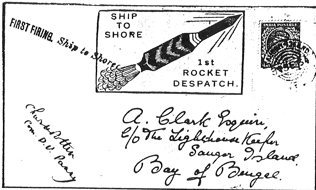
□ Fig. E: I 30-årene sendte Stephen Smith opp en rekke postraketter i India og Sikkim. Dette brevet er fra hans første rakett oppskutt nær Calcutta 30. september 1934.
