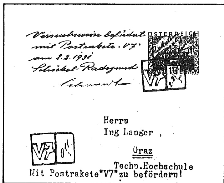
□ Fig. D: Et av de 102 brevene som ble sendt med Schmiedls postrakett V7 den 2. februar 1931 fra Schoekel til Radegund i Østerrike.
