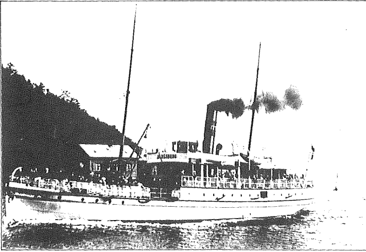
Fig. 127. Dampskipet «Yrjar» (Nr. 1) den tid det het «Jarlsberg». Etter Olaf T. Engvig.
