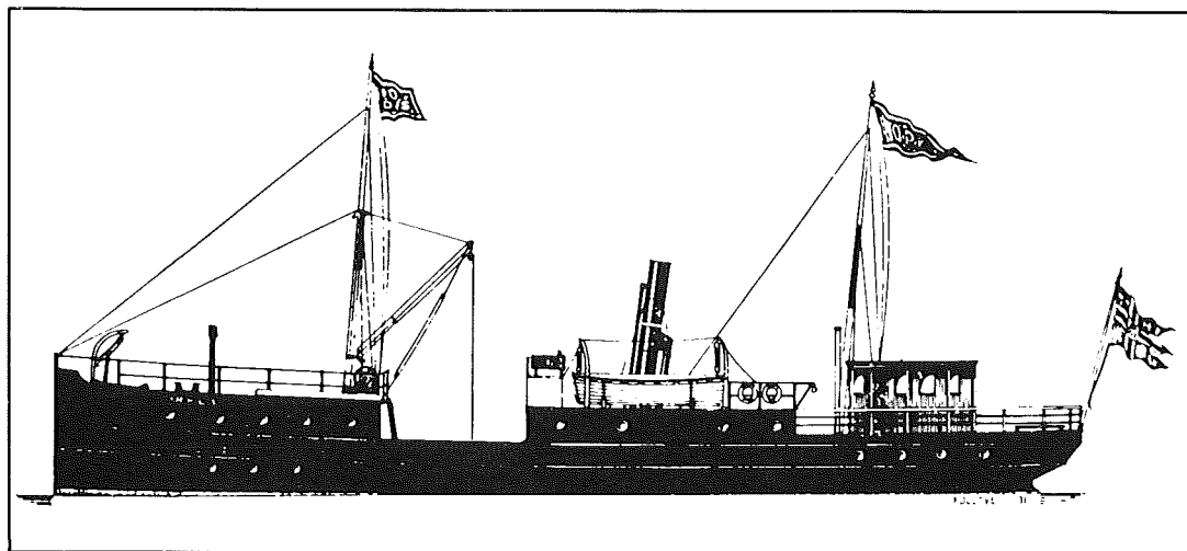
Fig. 56. Dampskipet «Orkla» (Nr. 1), tegnet av konservator Bård Kolltveit. Etter Olaf T. Engvig.
