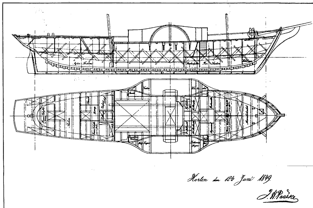
Fig. 3 Utsnitt av J. H. Paaskes tegninger til dampskipet «Nidelven». Etter Pedersen og Koren.
