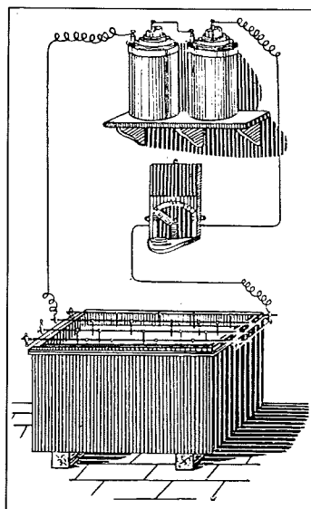
Fig. 3. Bildet viser et galvanisk bad for kobberutfelling med batterier som strømkilde og innkoblet spenningsregulator.
