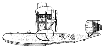
Fig. D: Supermarine Channel sjøfly benyttet på åpningsturene 12. og 13. juli 1920. Postverkets særstempler fra 1970 og 1980 til minne om åpningen viser et Lübeck—Travemünde, som ble satt inn noe senere.
