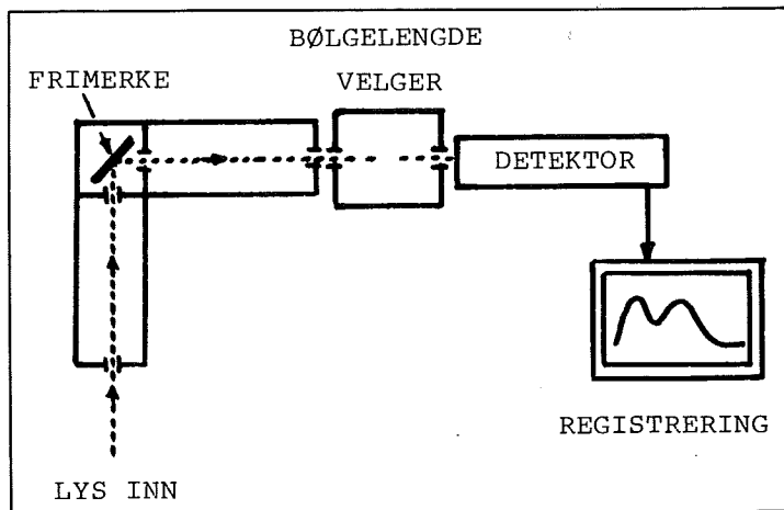
FIGUR 3. SKISSE AV MÅLEUTSTYR FOR LUMINESCENS-REGISTRERING. Et utstyr for studier av luminescens fra bl.a. frimerker, ses her ovenfra. Energirikt UV-lys blir sendt inn mot frimerket, og luminescenslys som sendes ut fra frimerket mot høyre blir undersøkt. Bølgelengden av interesse blir valgt ved hjelp av en bølgelengdevelger. Lysintensiteten blir målt ved en detektor og til slutt registrert.
