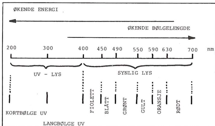
FIGUR 2. ENERGI OG BØLGELENDE HOS LYS. Bølglengden er gjengitt i nanometer (nm) som er en milliontedels mm. Bølglengde-intervallene for spekterets forskjellige farger er også merket av.
