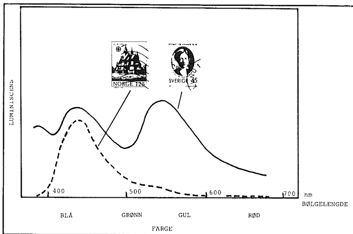
FIGUR 4. LUMINESCENS FRA TO FORSKJELLIGE FRIMERKER. Registreringene er tatt opp med et utstyr som i figur 3, og en ser at de to kurvene er helt forskjellige — luminescensen har ikke samme fargesammensetning for de to frimerkene. (Bølgelengde i nm og tilsvarende farge er merket av ved den horisontale aksen.)
