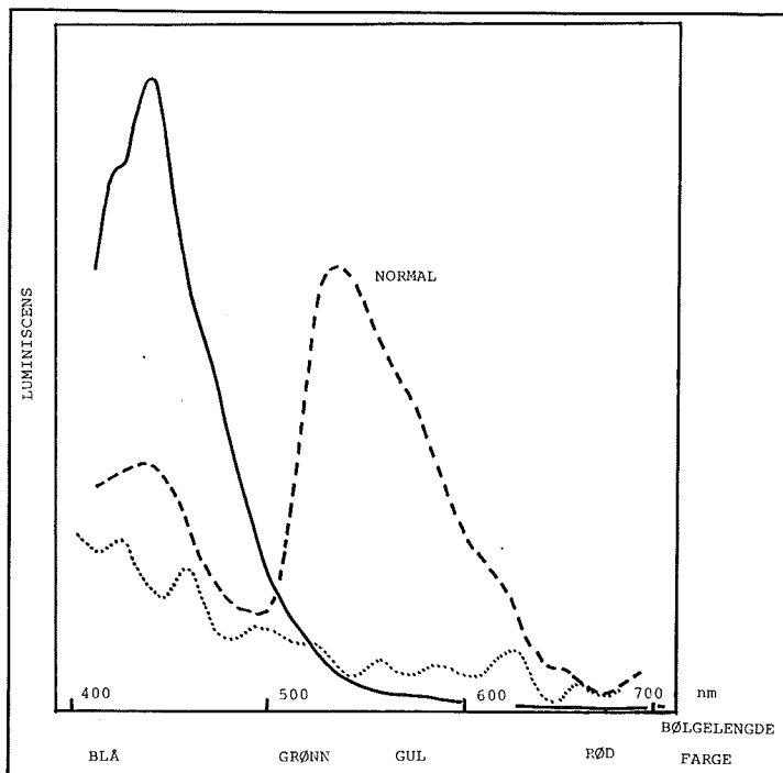
FIGUR 7. SPEKTRALMÅLINGER PÅ FRIMERKENE I FIGUR 6. Luminescensen fra de tre frimerkene i figur 6 er helt forskjellig. Stiplet linje viser normal luminescens fra dette frimerke (det venstre i figur 6). Punktert linje viser den lave gjenstående luminescensen til frimerket i midten av figur 6. Heltrukket linje viser spektrum til luminescensen fra frimerket til høyre i figur 6 (med blekemiddel).
