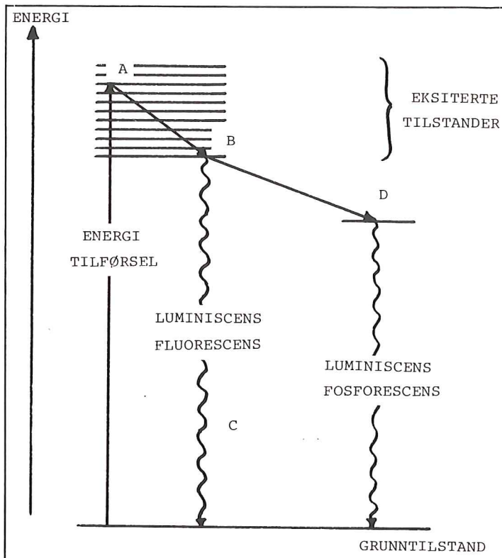
FIGUR 1. HVORDAN OPPSTÅR LUMINESCENS? Tilførsel av energi kan løfte et molekyl fra hviletilstanden «grunntilstanden». Molekylet kommer da til energinivået A og er «eksitert». Deretter går molekylet til B, og kan derfra ofte gå to veier: enten til C eller D. Første muligheten, C, gir opphav til luminescens i form av fluorescens. Den andre muligheten, D, betyr at molekylet kommer i en såkalt metastabil tilstand. Det kan nå oppstå luminescens ved at molekylet går tilbake til hviletilstanden. Denne senere form av luminescens blir kalt fosforescens.
