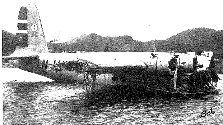
Fig G: DNL's Sandringham LN-IAW «Bukken Bruse» etter hevingen ved Hommelvik.
