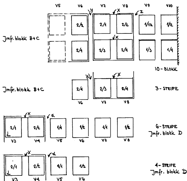
Fig. 6. Typiske rammeformer x-y-z-d.
