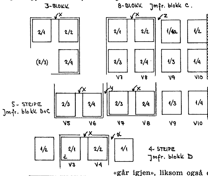
Fig. 7. Typiske rammeforhold x-y-z-d.
