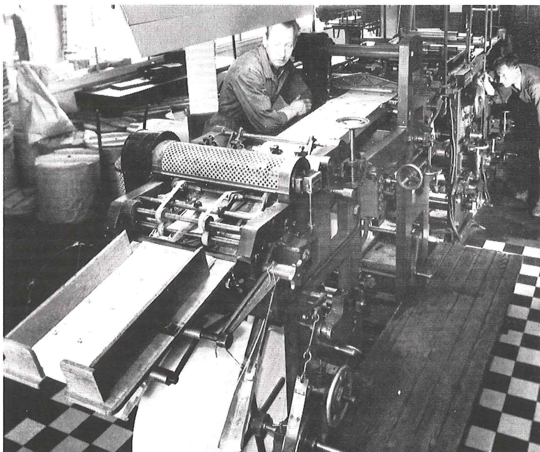
Dypptrykkspressen fra Goebel i Darmstadt var i uavbrutt virksomhet med trykking av frimerker og helsaker fra 1936 frem til 1974. Bildet er tatt i 1958.
