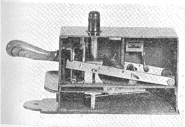
Fig. 3. Maskinen i forskjellige stillinger.
