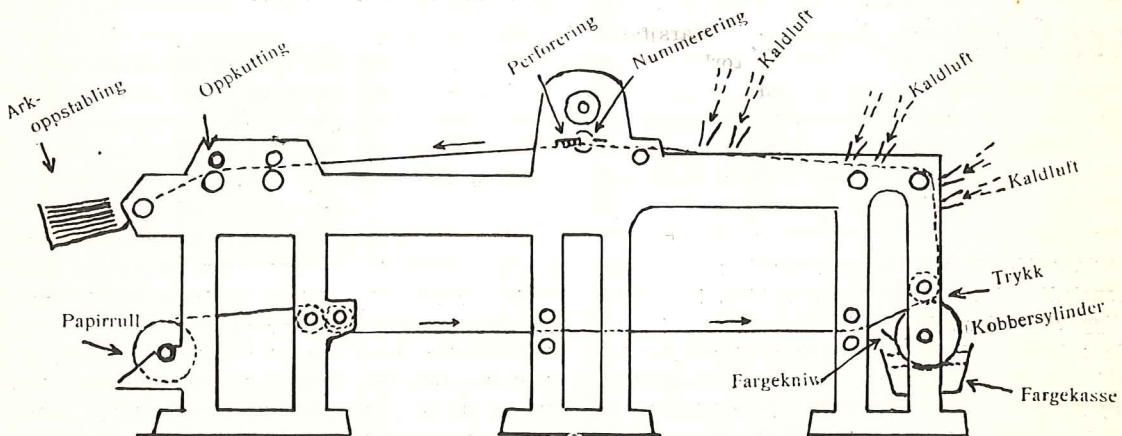
Fig. 3. Skjematisk skisse av maskinen.
